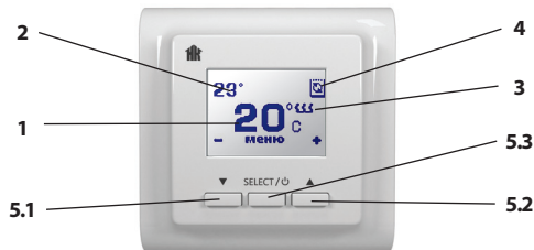
Рис. 2 Главная индикация в основном режиме работы
