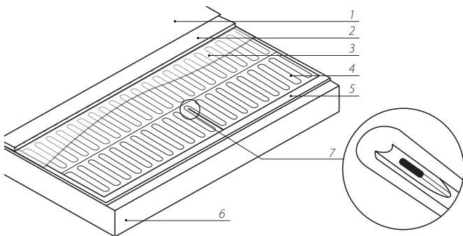
Рисунок 7. Конструкция элементов пола с использованием в качестве финального покрытия линолеума или коврового покрытия
