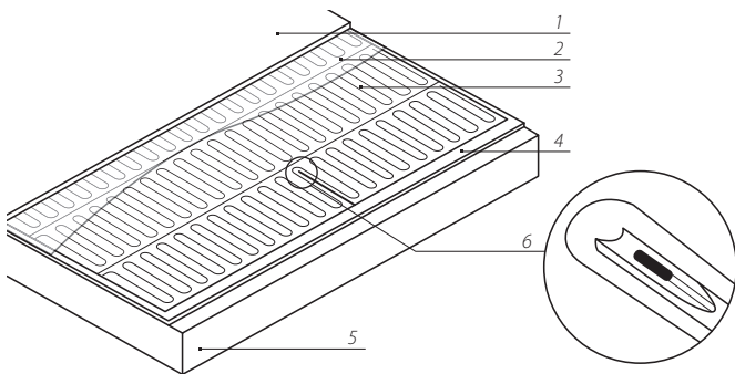
Рисунок 6. Конструкция элементов пола с использованием в качестве финального покрытия ламината или паркетной доски
